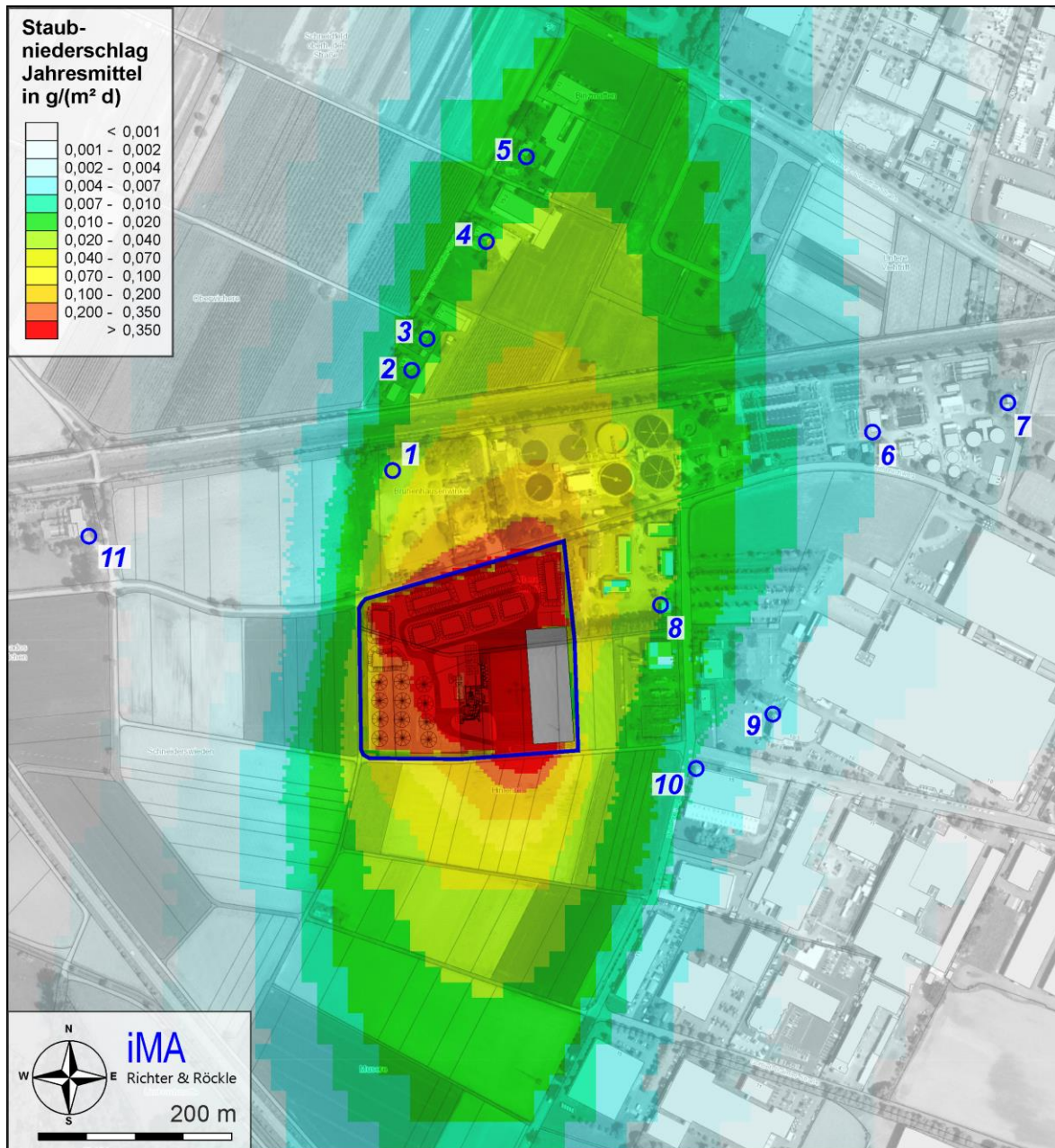
Abbildung 7-5: Staubniederschlag: Jahresmittelwerte des Immissionsbeitrags der Asphaltmischanlage und der Recyclinganlage. Irrelevanzschwelle: 0,0105 g/(m²·d); Immissions(grenz)wert: 0,35 g/(m²·d)
