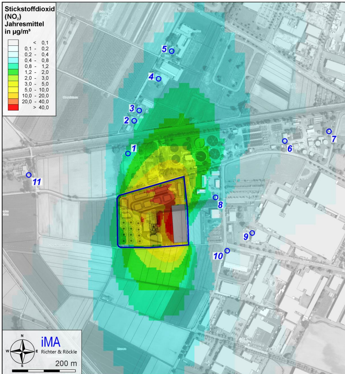
Abbildung 7-6: NO 2 : Jahresmittelwerte des Immissionsbeitrags der Asphaltmischanlage und der Recyclinganlage. Irrelevanzschwelle: 1,2 µg/m 3 ; Immissions(grenz)wert: 40 µg/m 3
