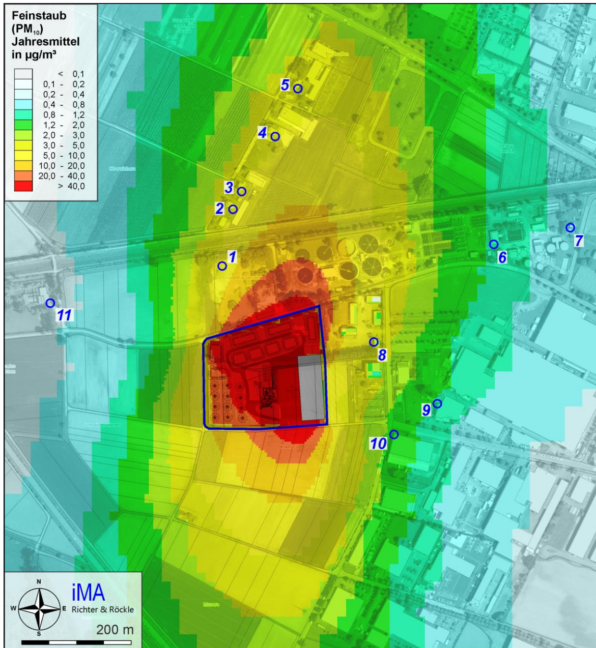
Abbildung 7-3: PM 10 : Jahresmittelwerte des Immissionsbeitrags der Asphaltmischanlage und der Recyclinganlage. Irrelevanzschwelle: 1,2 µg/m 3 ; Immissions(grenz)wert: 40 µg/m 3
