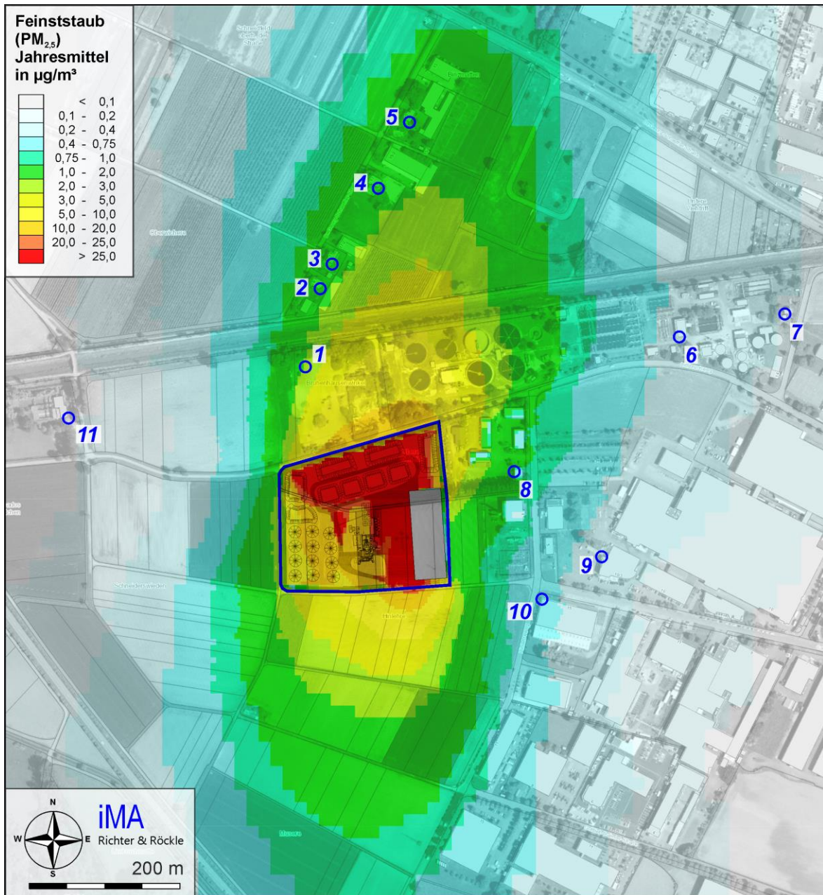
Abbildung 7-4: PM 2,5 : Jahresmittelwerte des Immissionsbeitrags der Asphaltmischanlage und der Recyclinganlage. Immissions(grenz)wert: 25 µg/m 3
