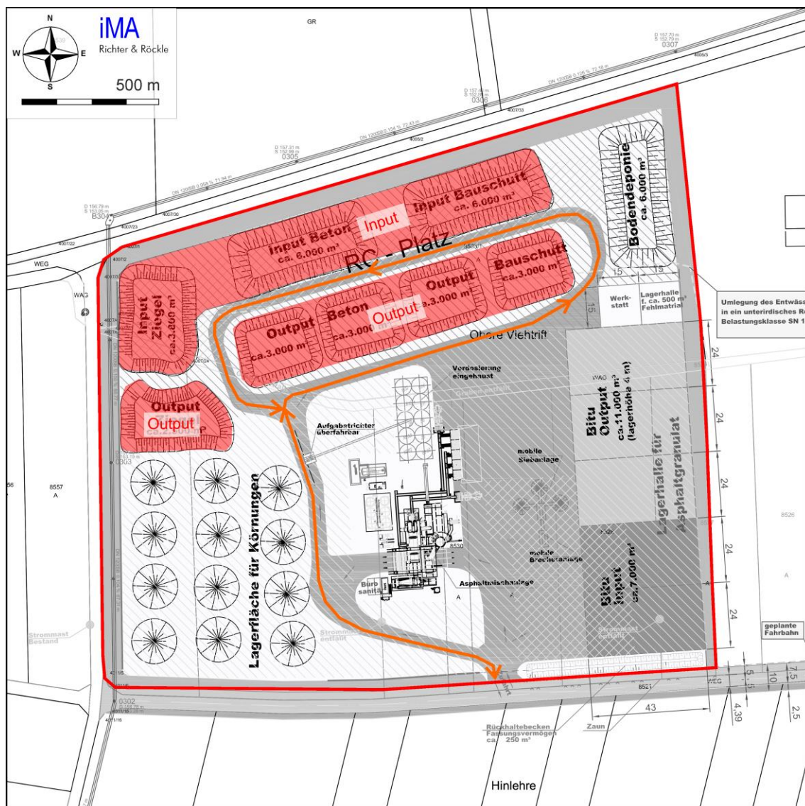
Abbildung 4-2: Plan der Recyclinganlage und der Fahrwege (schematisch).
