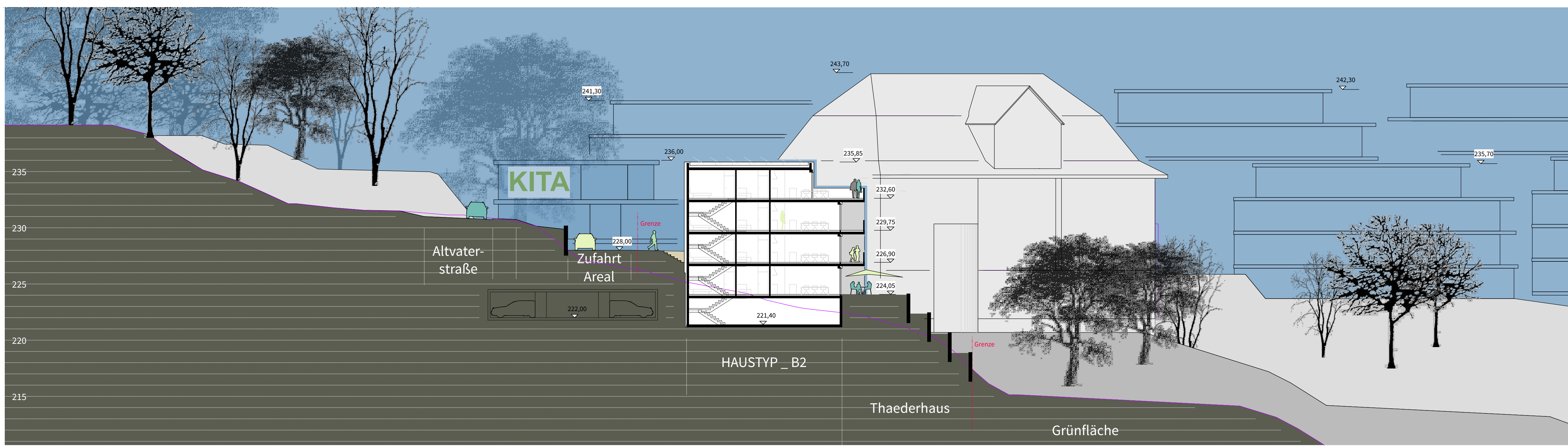
Schnitt 01
