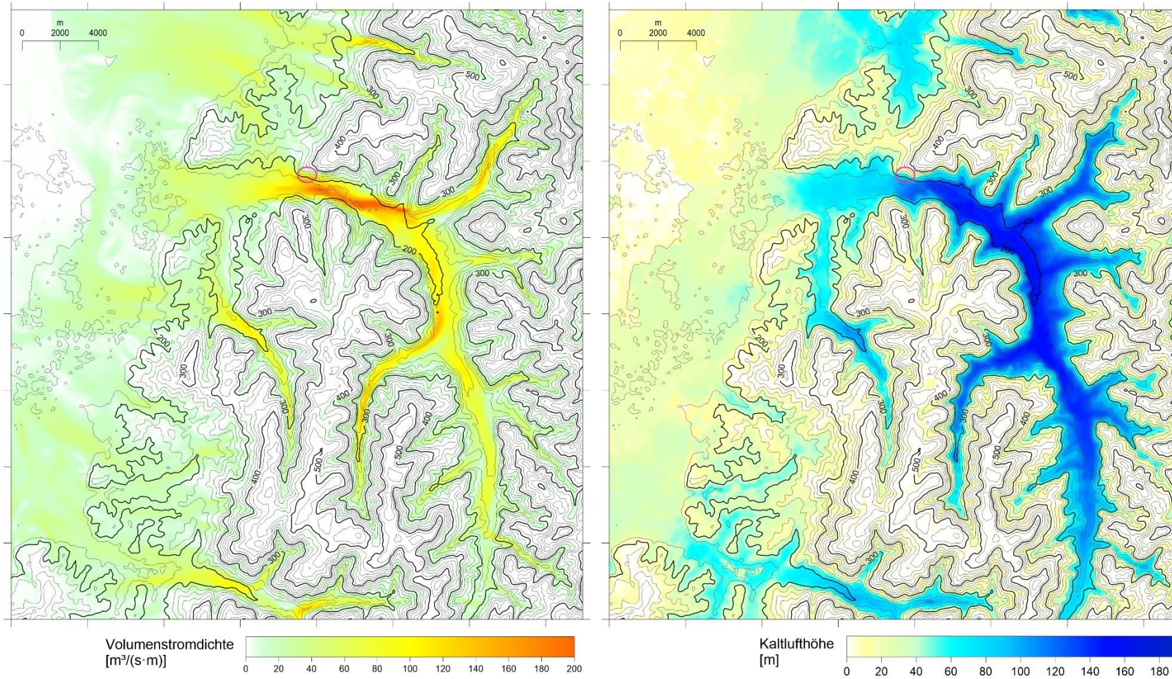
Abbildung A-2: Volumenströme (links) und Kaltluflhöhen (rechts) zu im weiteren Verlauf der Nacht (2 Stunden nach Einsetzen der Kaltluftabflüsse).
