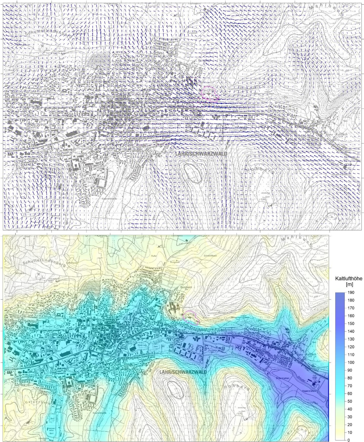
Abbildung A-5: Mittlere Windgeschwindigkeiten 2 Stunden nach Einsetzen der Kaltluftabflüsse (oben) und Höhe der fließenden Kaltluft (unten).
