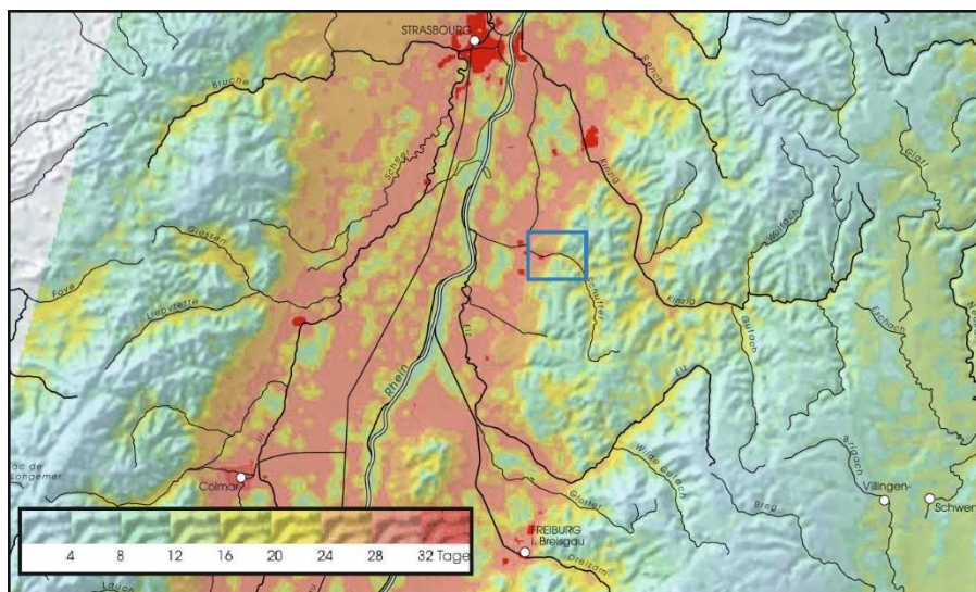
Abbildung 4-1: Tage mit Wärmebelastung (aus REKLIP-Atlas, 1995)
