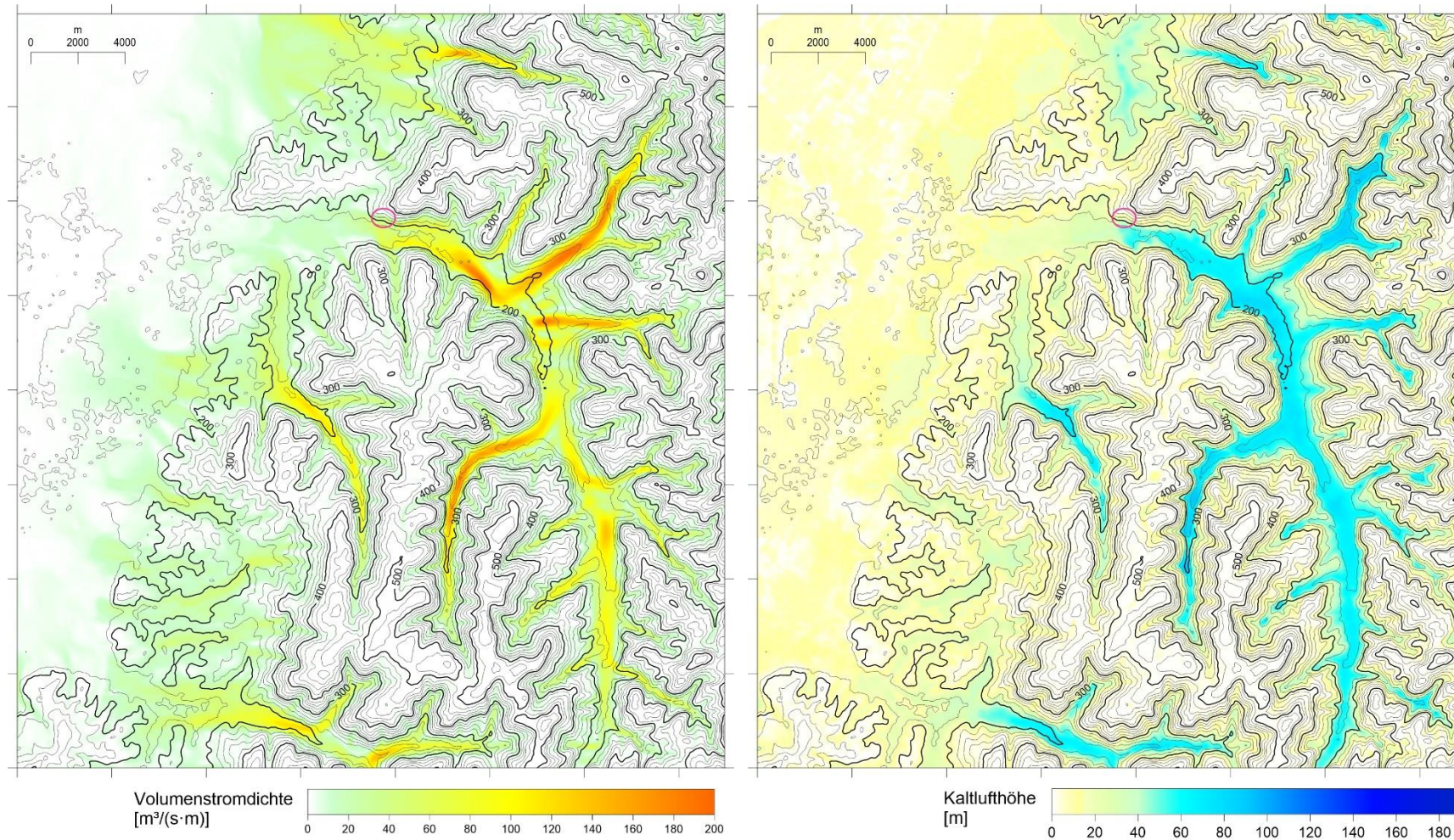
Abbildung A-1: Volumenströme (links) und Kaltluflhöhen (rechts) zu Beginn der Nacht (1 Stunde nach Einsetzen der Kaltluftabflüsse).
