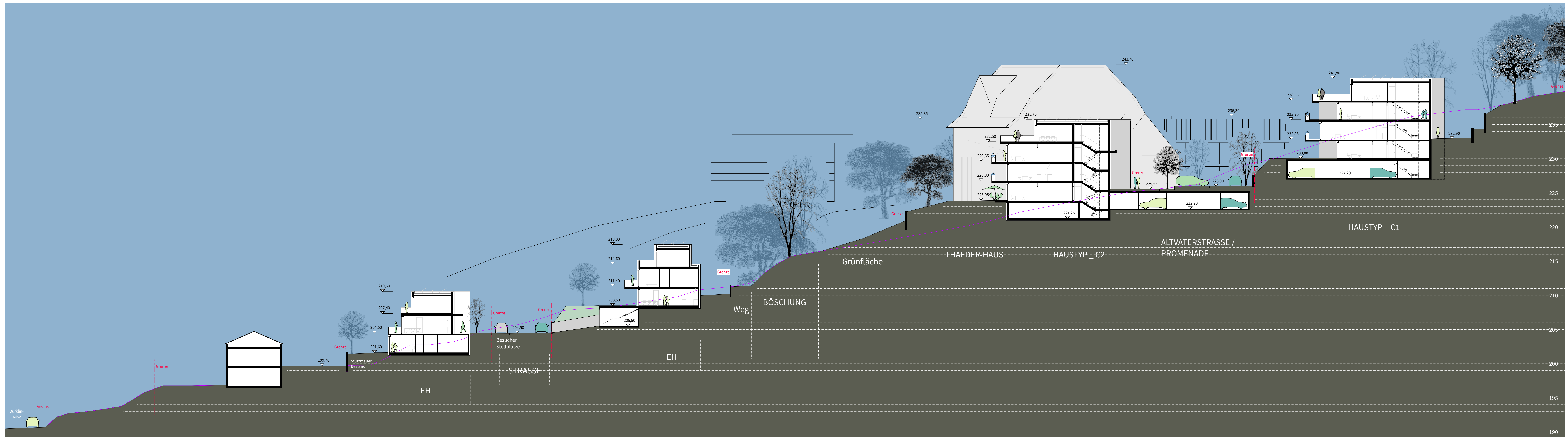
Schnitt 04
