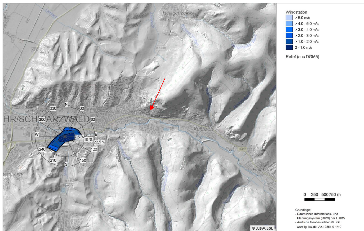
Abbildung 4-2: Gemessene Windverhältnisse in Lahr (LUBW-Station, 1991-1992). Das Plangebiet ist durch einen Pfeil gekennzeichnet.
