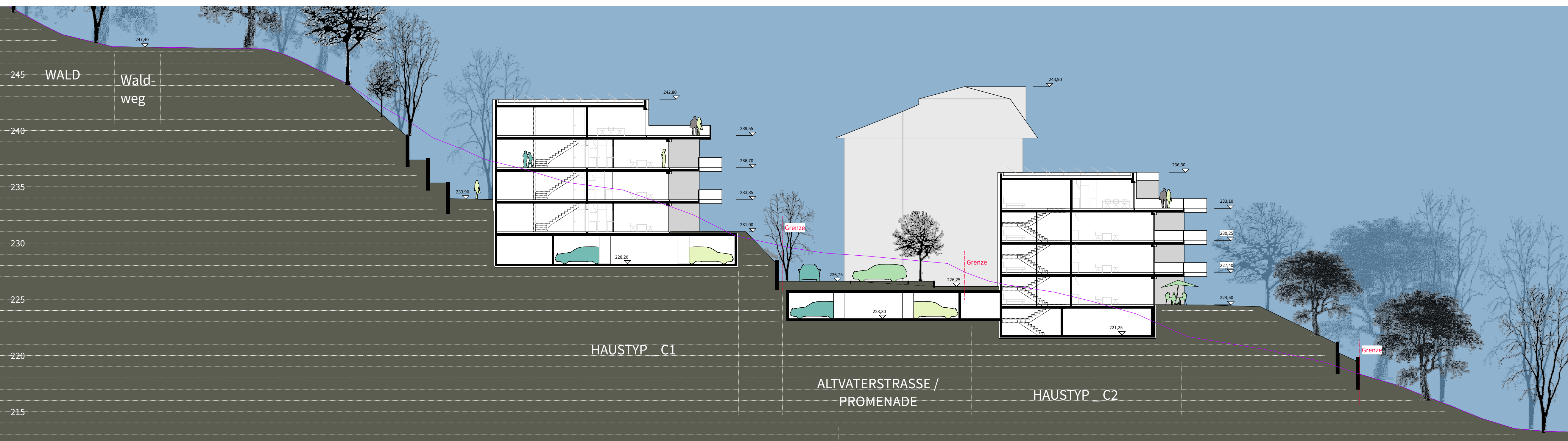
Schnitt 06
