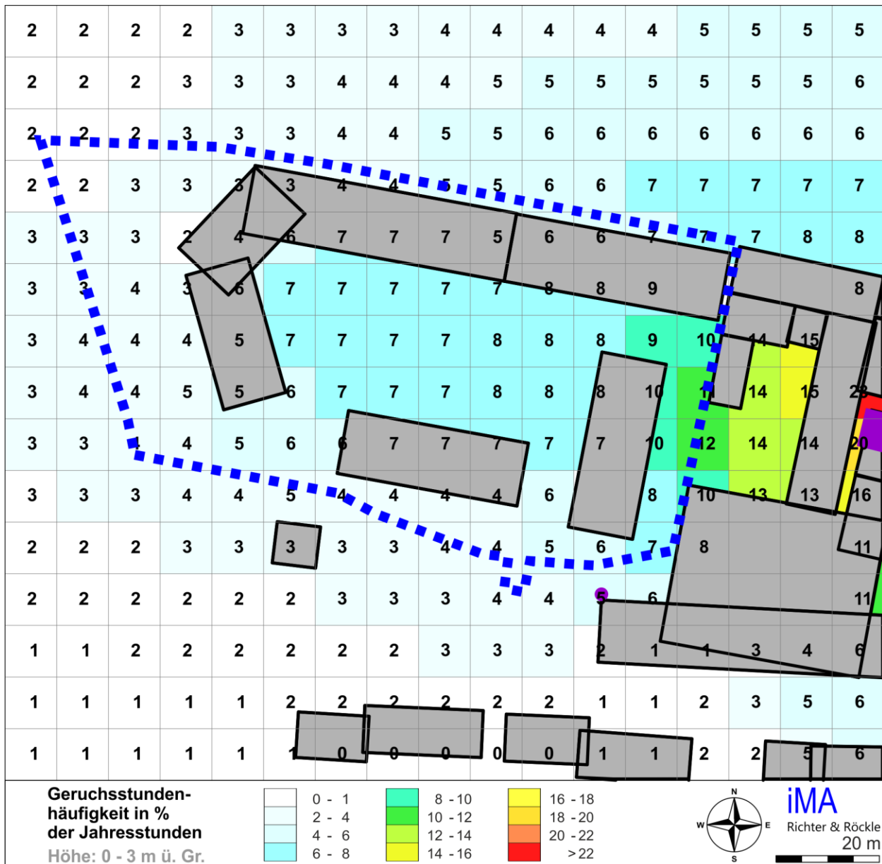
Abbildung A1-12: Geruchsimmissionsbeitrag der Fa. Padberg in der Höhenschicht 0 – 3 m bei einer Schornsteinhöhe zur Ableitung der Fortluft aus der Lackieranlage und der Fortluft aus der Edelstahl-Schweißerei von 18,5 m über Grund (Planfall 2). Dargestellt ist die relative Häufigkeit von Geruchsstunden pro Jahr in Prozent. Das Bebauungsplangebiet ist blau gestrichelt umrandet und enthält die geplante Bebauung. Die Emissionsquellen sind violett markiert. Die im Modell berücksichtigten Gebäude sind dunkelgrau umrandet. Die Gebäude, die in die Höhenschicht 0 m – 3 m hineinragen, sind grau hinterlegt. Derzeitige Emissionen.
