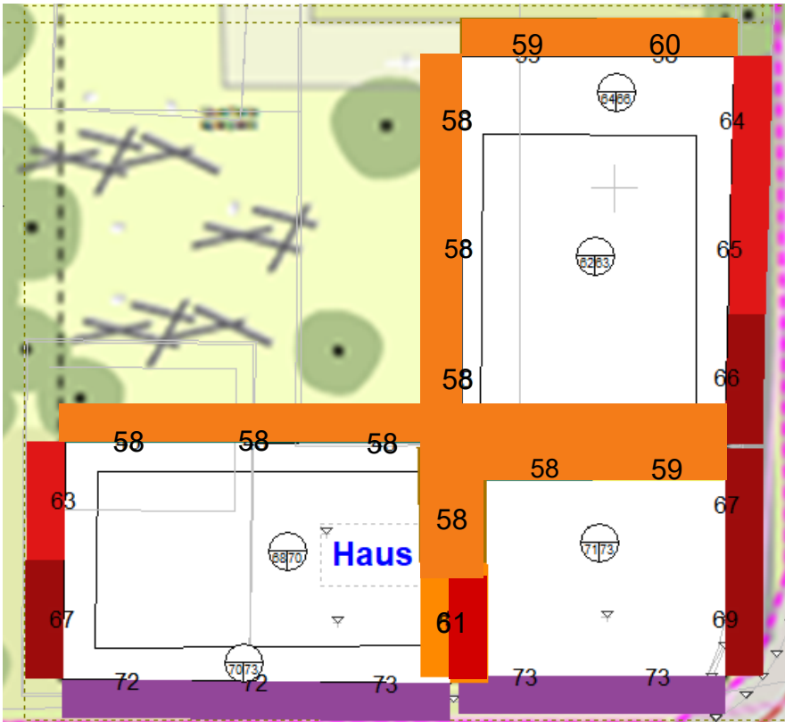
Abbildung 10: Maßgeblicher Außenlärmpegel Haus 1, 3. Obergeschoss
